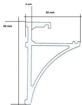
Glasplattenträger - Profil Supra 2
